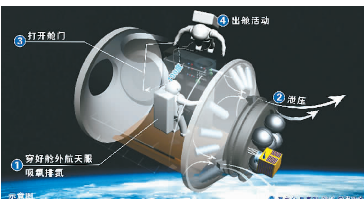
神七航天员出舱活动示意图
