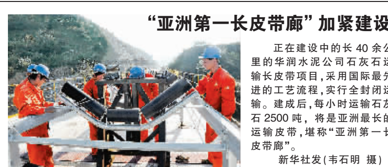
正在建设中的长 40 余公里的华润水泥公司石灰石运输长皮带项目, 采用国际最先进的工艺流程, 实行全封闭运输。建成后, 每小时运输石灰石 2500 吨, 将是亚洲最长的运输皮带, 堪称“亚洲第一长皮带廊”。 新华社发 (韦石明 摄)
