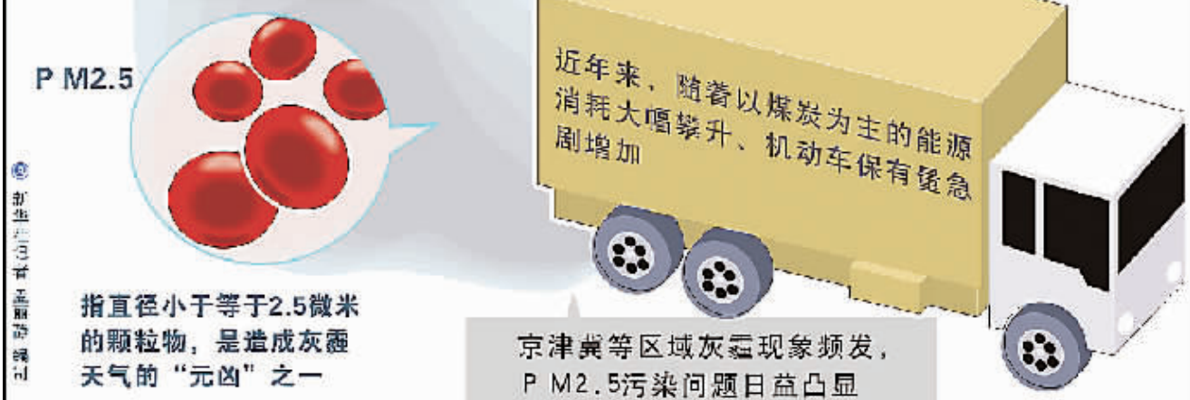
指直径小于等于2.5微米的颗粒物,是造成灰霾天气的“元凶”之一 京津冀等区域灰霾现象频发,PM2.5污染问题日益凸显
