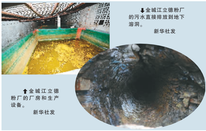
金城江立德粉厂的污水直接排放到地下溶洞。
