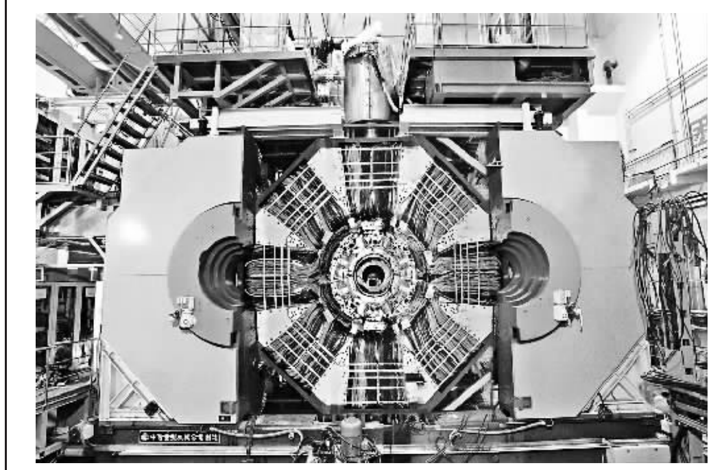
安装完成的北京谱仪 III。 新华社发
