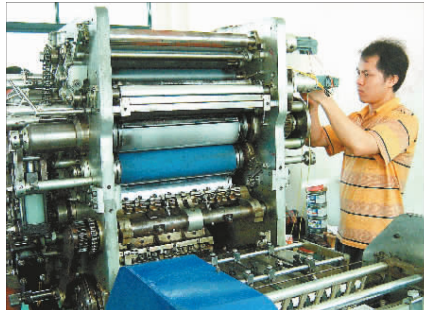
技术人员正在调试陈名乔发明的第一台虹式四色胶印机。 本报记者 程范滢 摄
