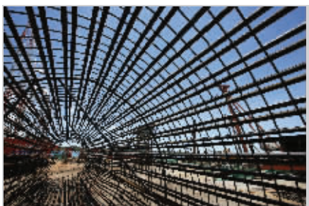
建设中的清澜大桥主墩
