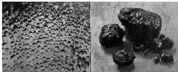
海底锰结核
