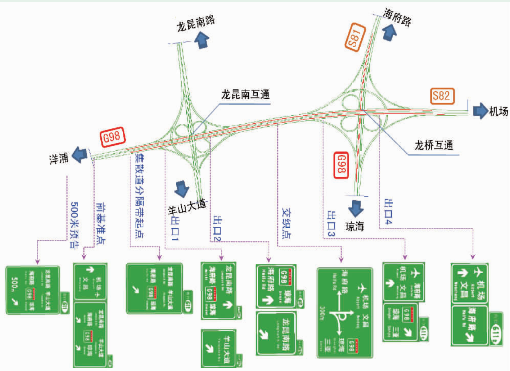
图2 从洋浦往机场方向标志布置示意图
