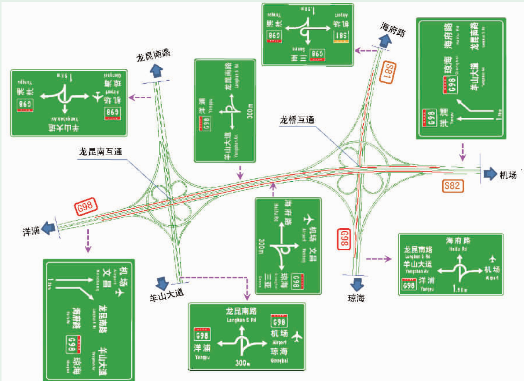
图8 龙桥、龙昆南互通图形化指路标志
