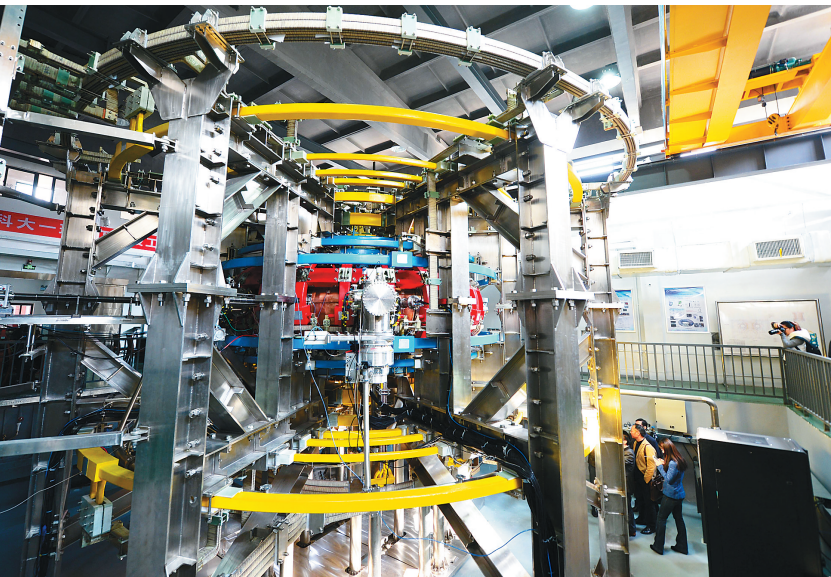
这是已进入常态化运行的大型反场箍缩磁约束聚变实验装置（11 月 3 日摄）。近日，我国首台大型反场箍缩磁约束聚变实验装置（KT-X，中文简称“科大一环”），在中国科学技术大学完成安装调试并进入常态化运行。据项目工程总指挥、中科大物理学院刘万东教授介绍，KT-X 是中国完全自行设计、自主研制集成的国际先进反场箍缩装置。它的建成将为国内外从事等离子体物理研究的科研人员提供一个全新的大型实验平台，对中国磁约束聚变领域高端人才培养，发展磁约束聚变科学技术研究事业具有重要意义。 新华社记者 刘军喜 摄
