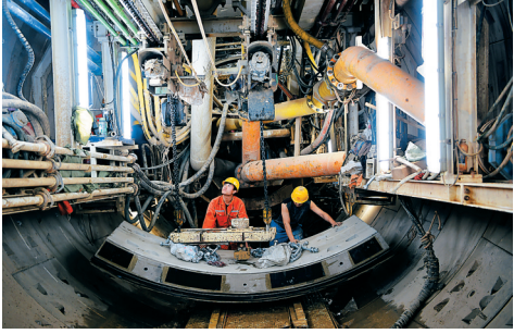
图为施工人员调运盾构管片准备衬砌隧道。 新华社记者 范培坤 摄
