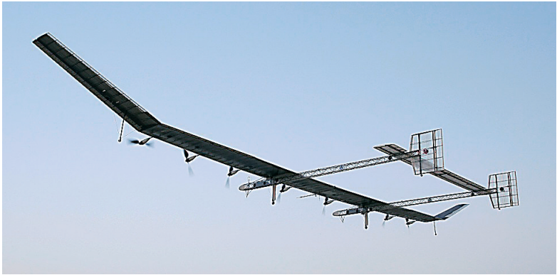
彩虹新型太阳能无人机在西北某机场试飞。 新华社发
