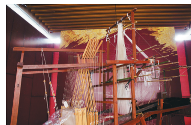
织锦机。
