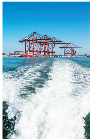
3 个 5 万吨级兼靠 2 个 10 万吨级小铲滩集装箱公共码头泊位已建成投用。
