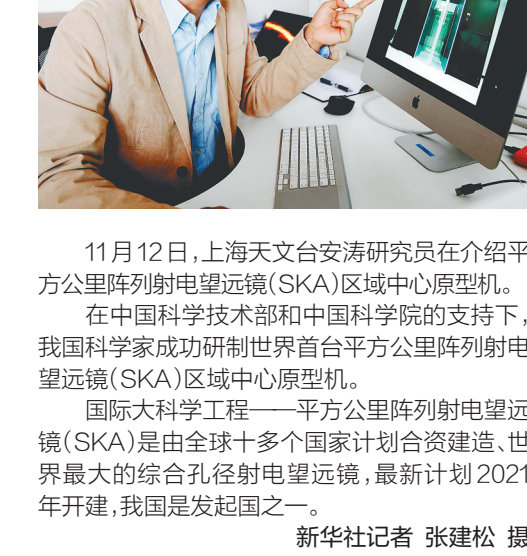
11月12日，上海天文台安涛研究员在介绍平方公里阵列射电望远镜(SKA)区域中心原型机。在中国科学技术部和中国科学院的支持下，我国科学家成功研制世界首台平方公里阵列射电望远镜(SKA)区域中心原型机。 国际大科学工程——平方公里阵列射电望远镜(SKA)是由全球十多个国家计划合资建造、世界最大的综合孔径射电望远镜，最新计划2021年开建，我国是发起国之一。 新华社记者 张建松 摄
