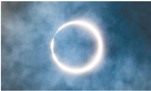
在西藏阿里拍摄的日环食(6月21日摄)。 新华社发(戴建峰 摄)
