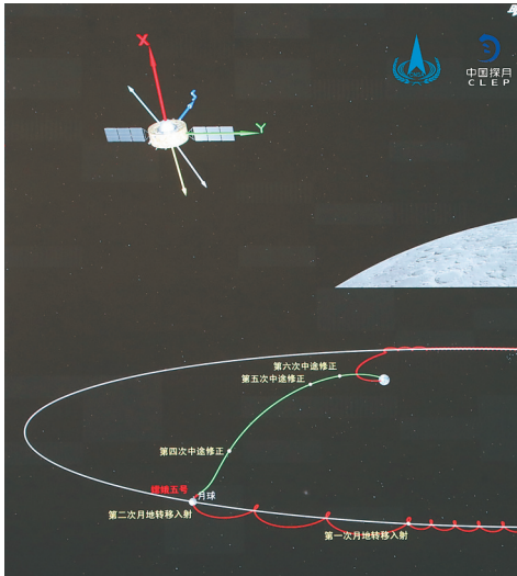
嫦娥五号轨道器和返回器组合体实施月地转移入射和中途轨道修正的示意图。新华社发
