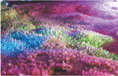
石花水洞聚宝盆——方解石晶花。 受访者供图
