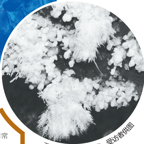
石花水洞中的文石花。受访者供图
