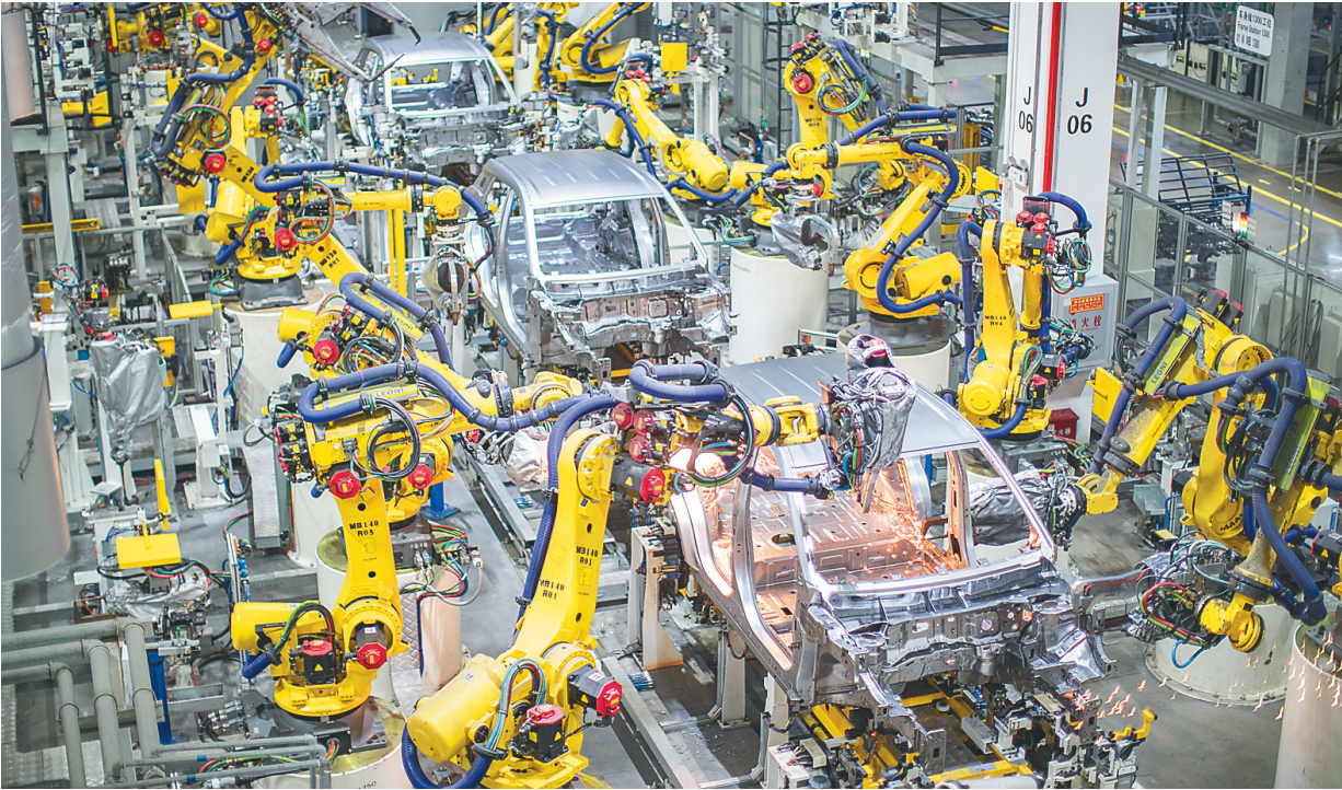
重庆一家新能源汽车企业使用智能化焊接机器人进行焊接作业。 新华社发
