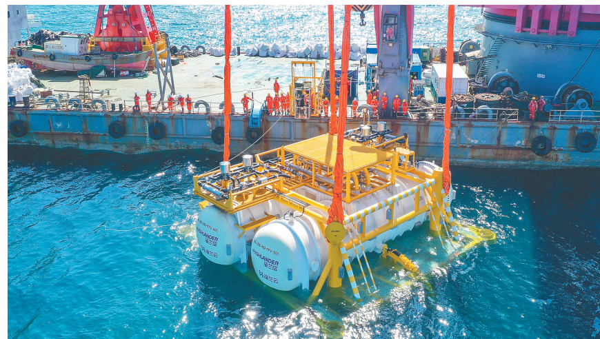
海南海底数据中心项目(一期)首舱下水施工现场。 通讯员 唐菲 摄
