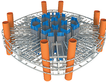
海南中心项目巨立柱。
