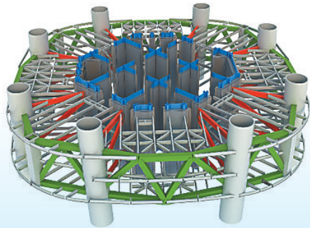
海南中心项目采取六道腰桁架+一道伸臂桁架结构。
