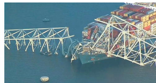
图为遭撞击后坍塌的“弗朗西斯·斯科特·基”大桥和撞击大桥的集装箱船。
