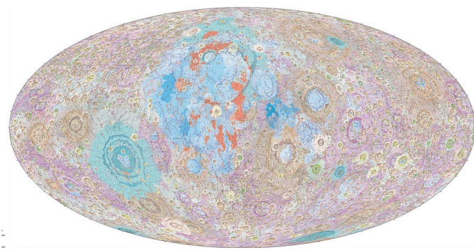
月球地质图。
