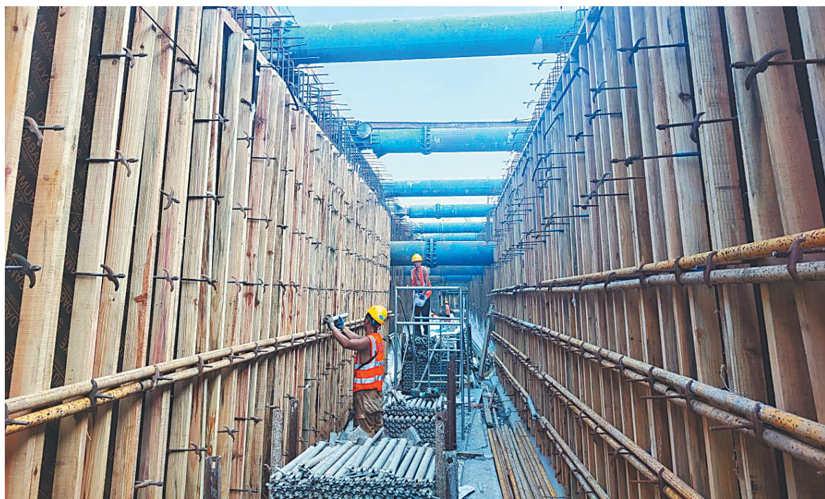
国庆期间,海口海文南路市政化改造工程项目现场,工人在有序施工。(项目部供图)
