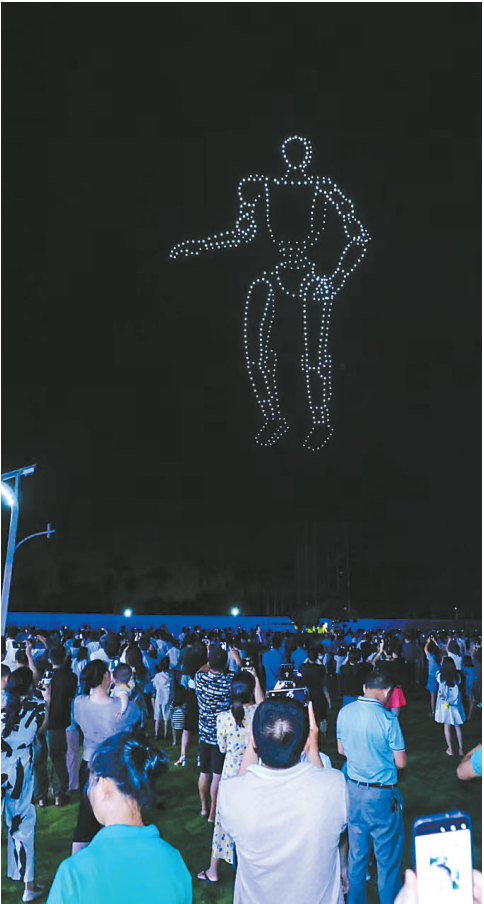
无人机表演。
