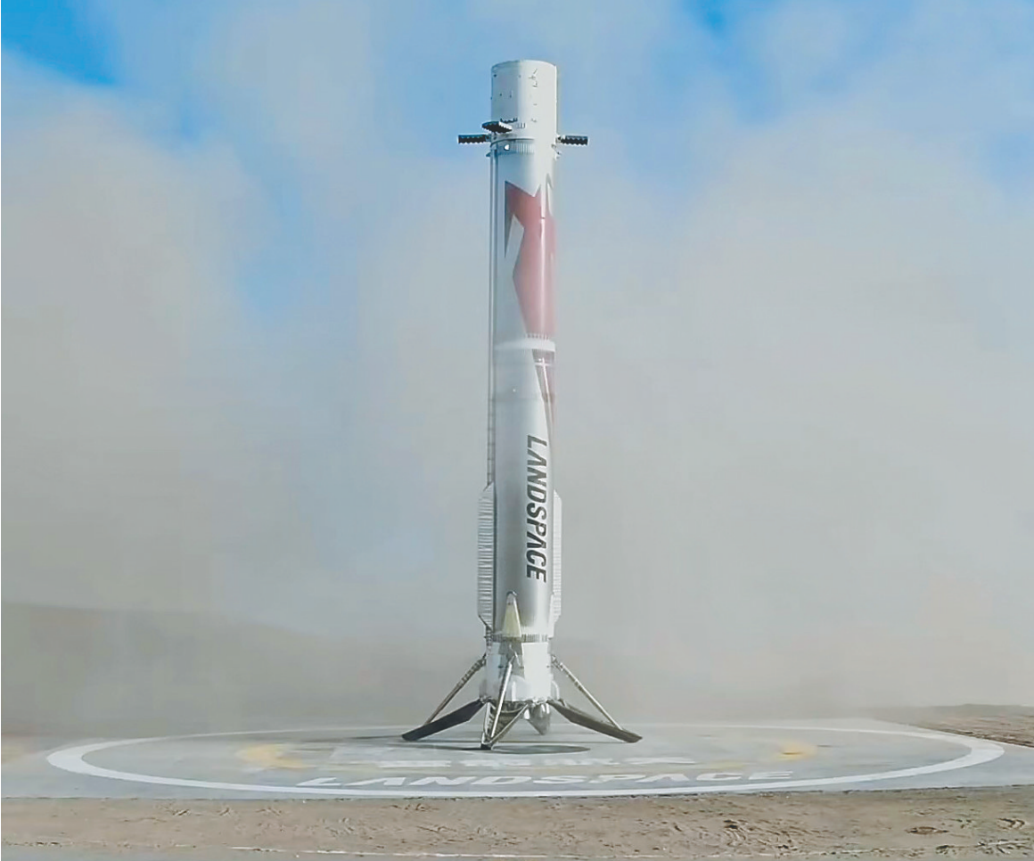
八月十九日,视频截图显示朱雀三号遥二运载火箭一子级按预定程序成功完成陆地回收。
